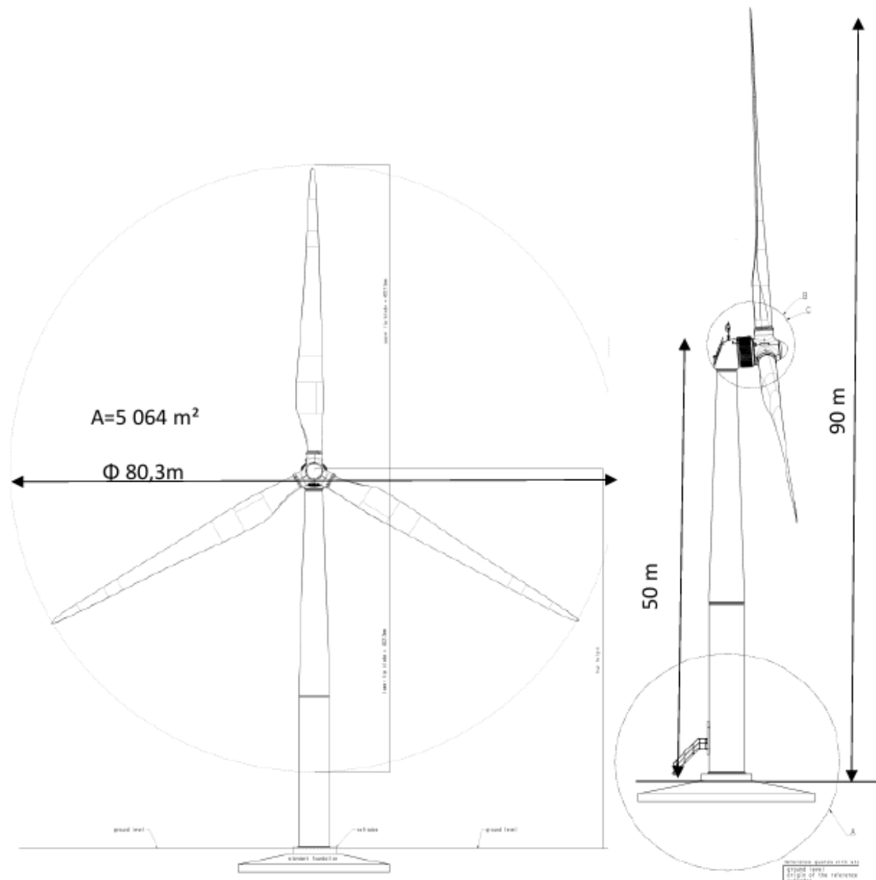
Figure 4 de la vue d'ensemble de l'éolienne LEITWIND LTW80 1650
